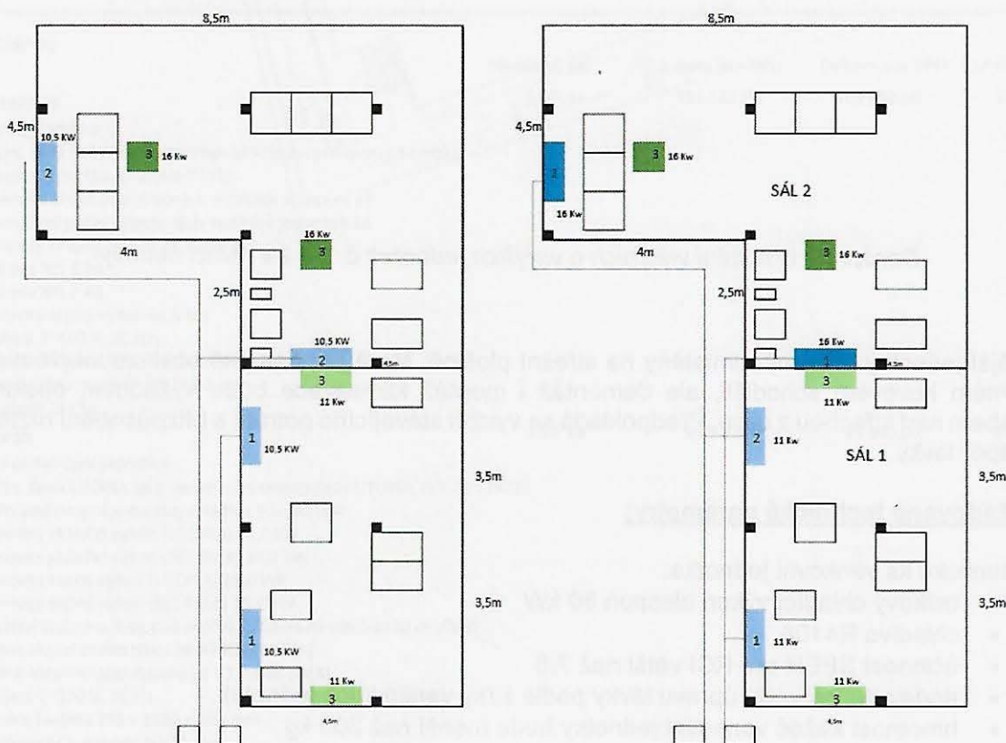
Obrázek 1 Stávající a stav (vlevo) a nově poptávaný stav (vpravo)
